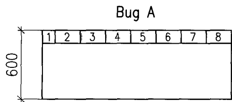
Рис. 18. Пример выполнения эскизного чертежа общего вида НКУ
